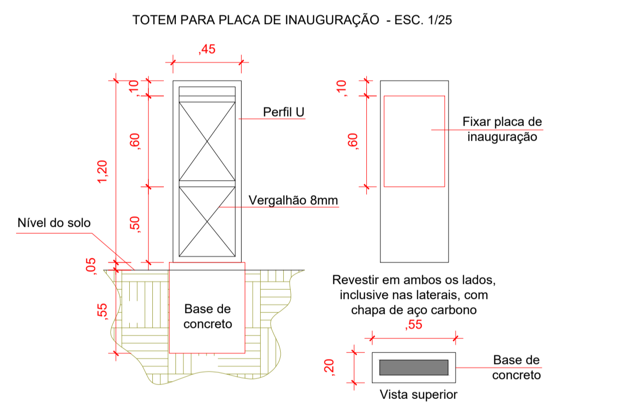
Corte AA
