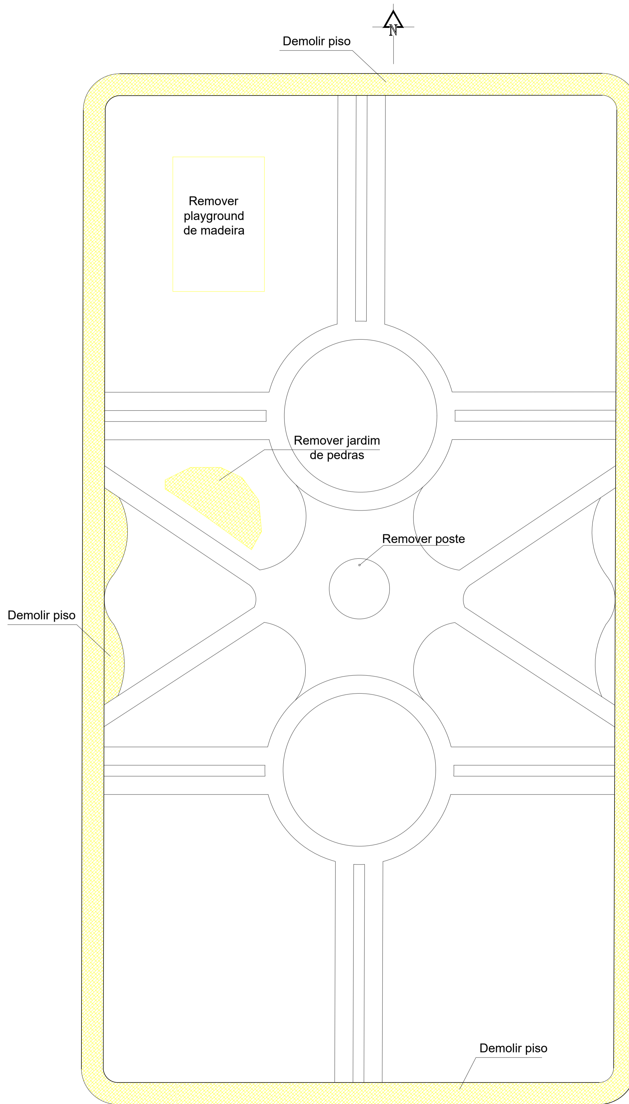
PLANTA - DEMOLIÇÕES ESC. 1:300
