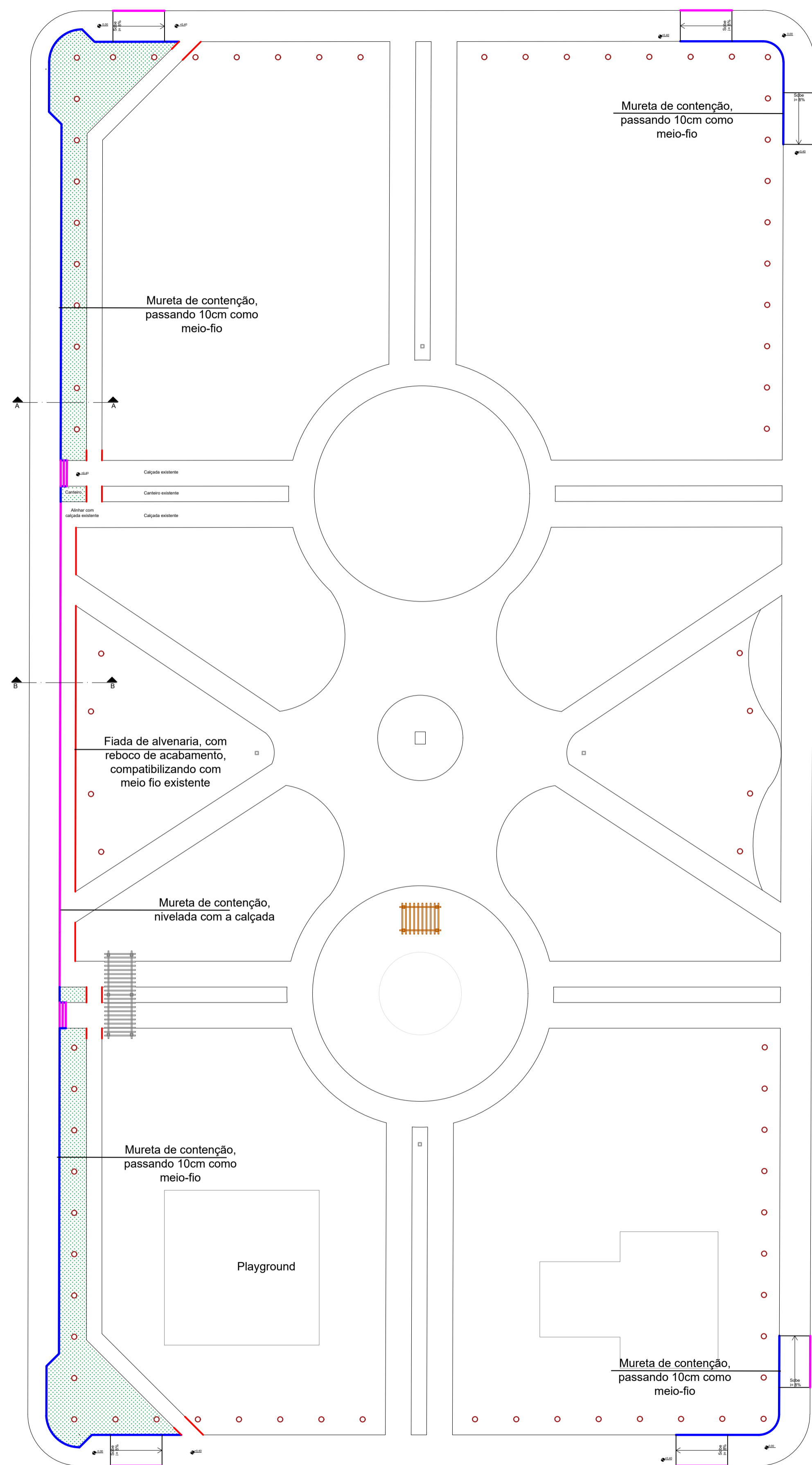
PLANTA - DETALHES MEIO-FIO ESC. 1:300
