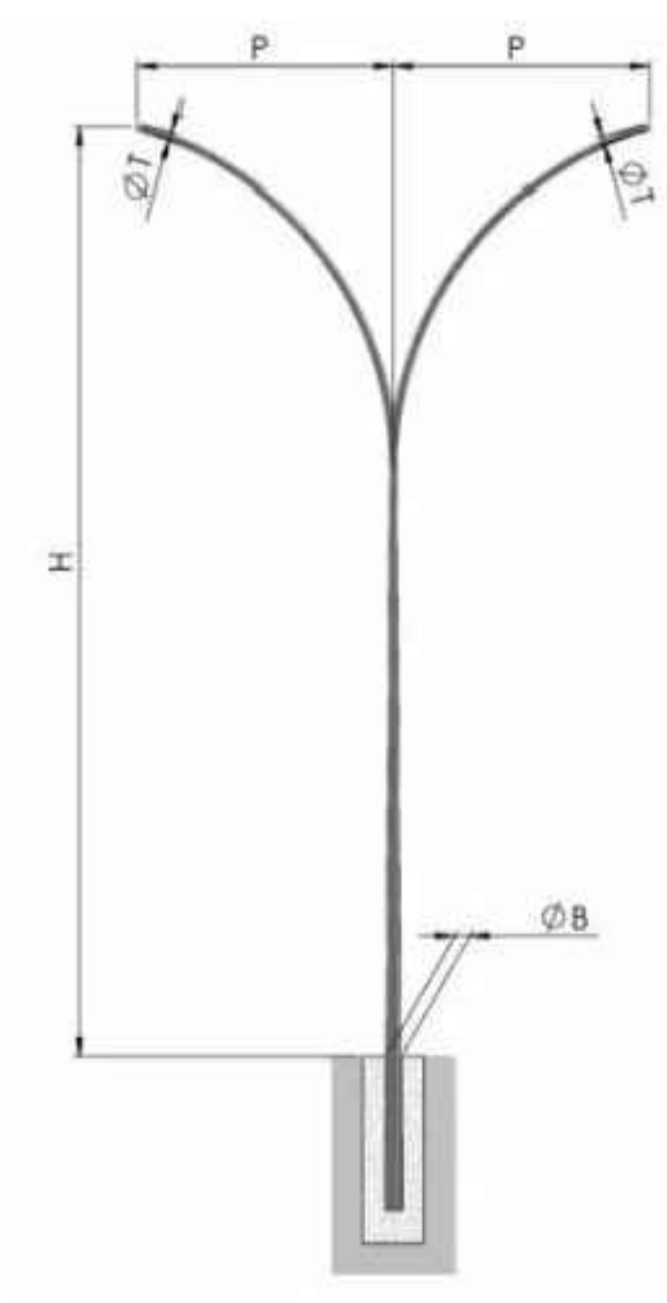
MODELO ILUSTRATIVO DO POSTE DE ILUMINAÇÃO S/ ESC.
