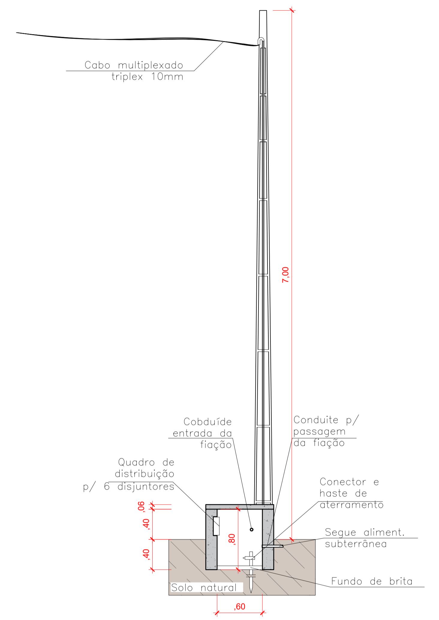
DET. CX. PASSAGEM 60X60 ESC. 1/30
