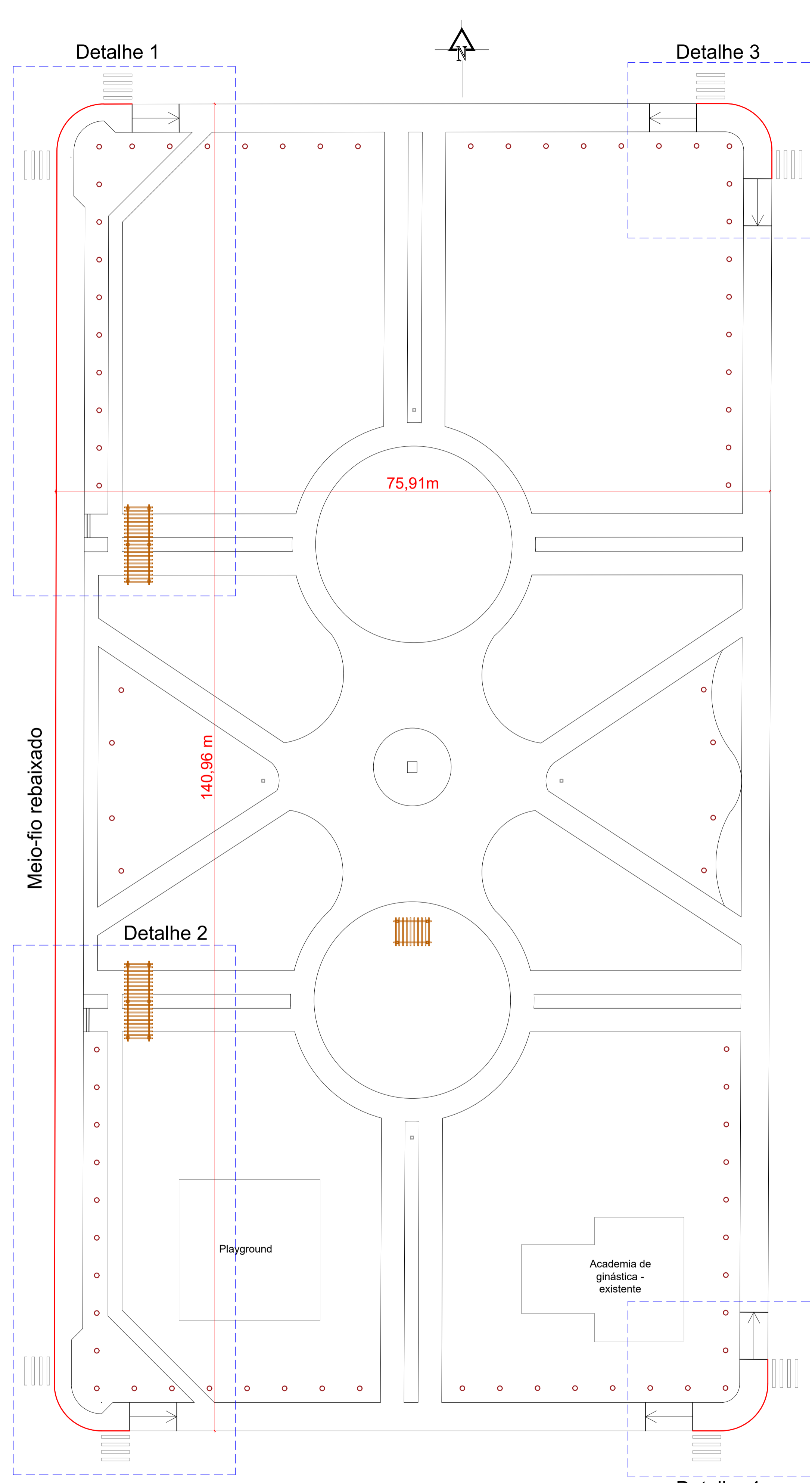
PLANTA - DETALHES ESC. 1:300
