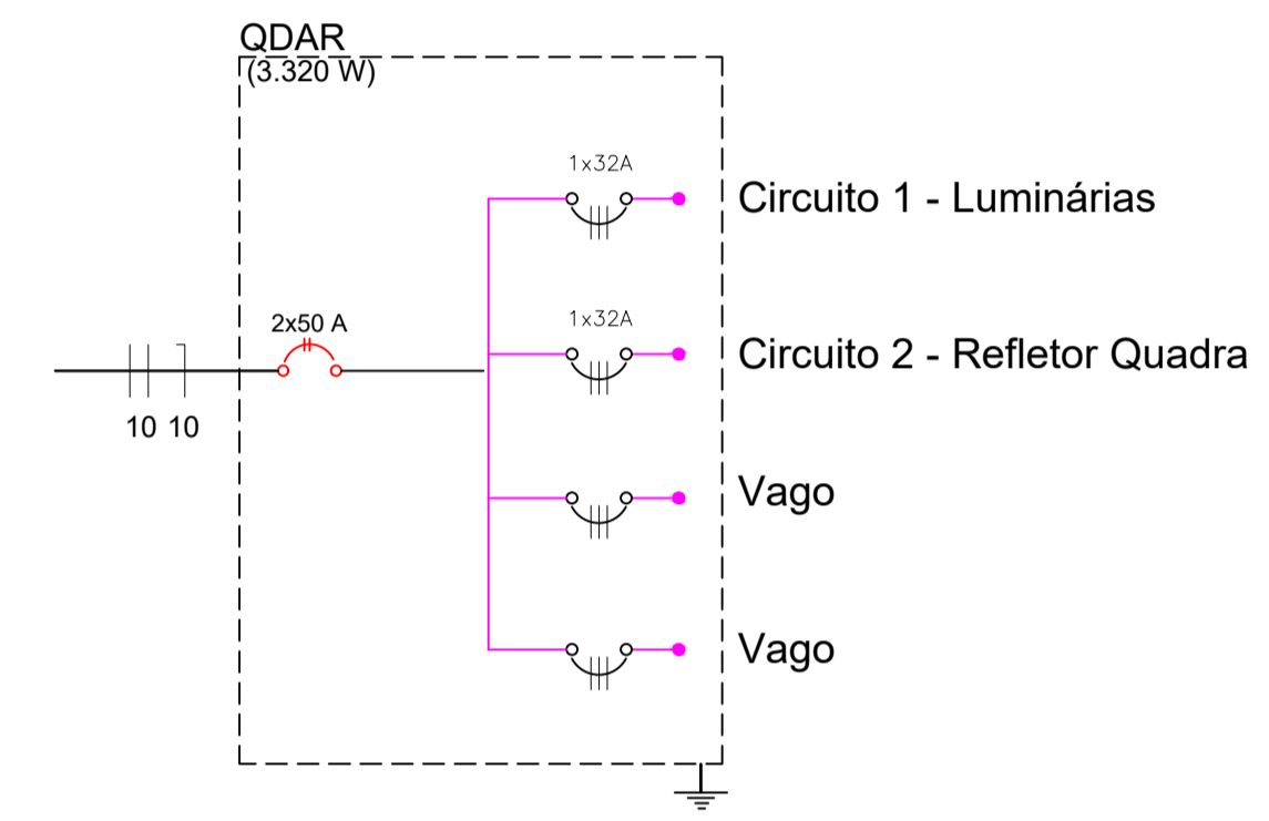
DIAGRAMA UNIFILAR S/ ESC.
