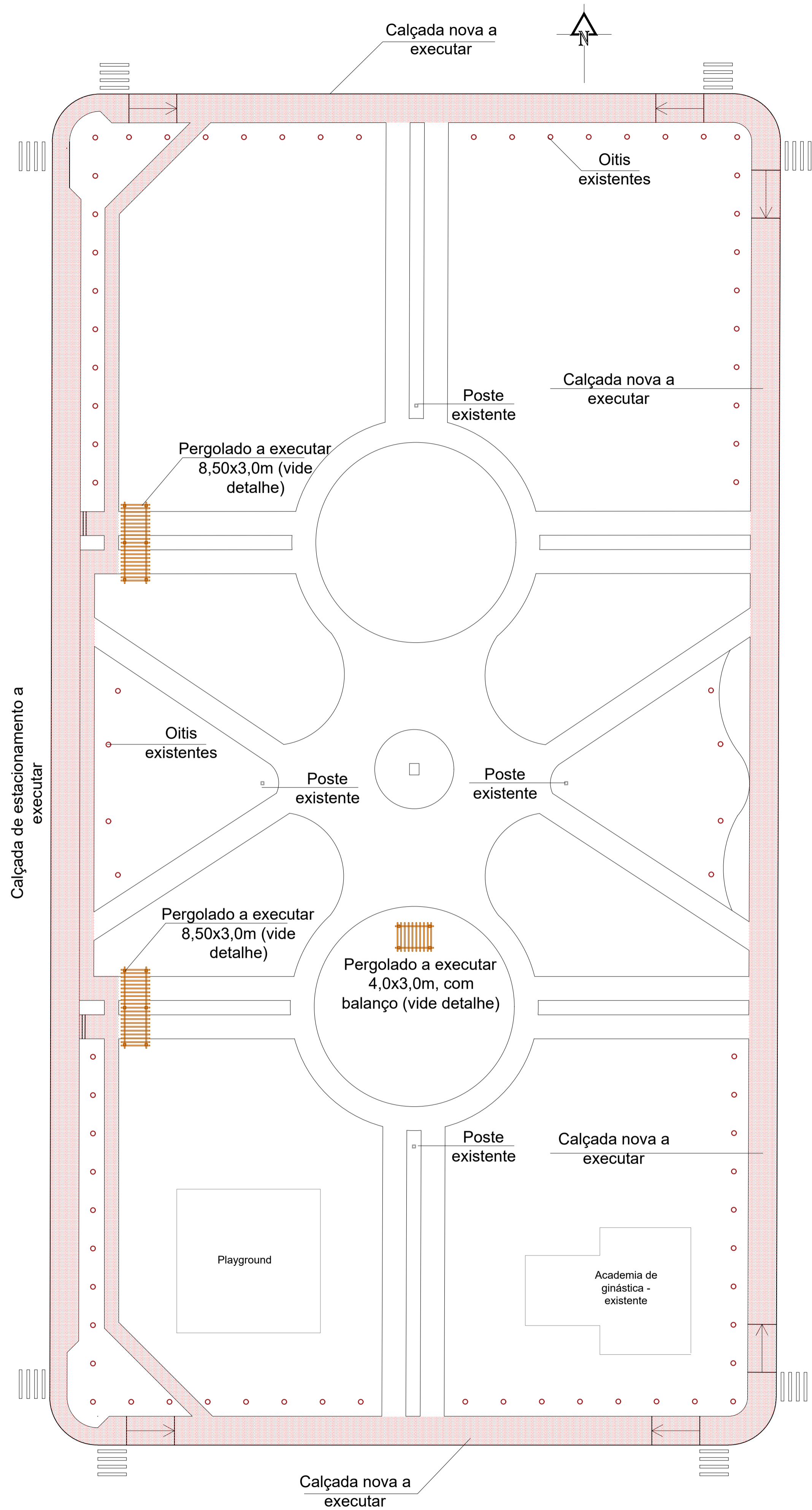
PLANTA - CONSTRUÇÃO DE CALÇADAS ESC. 1:300
