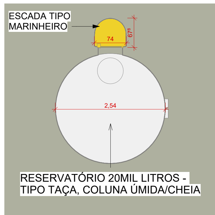
4 RESERVATÓRIO 1 : 50
