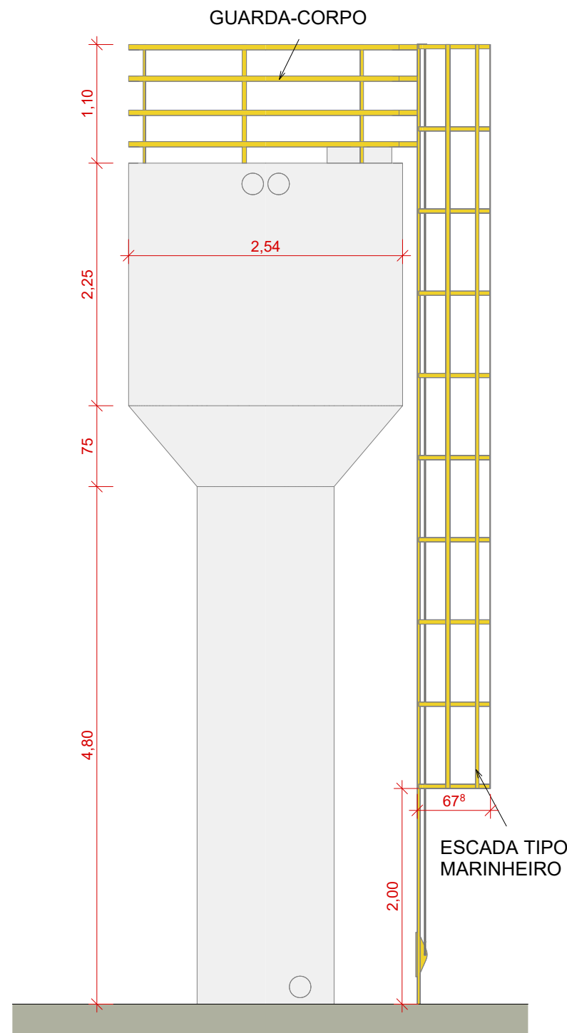
2 ELEVÇÃO ESQUERDA 1 : 50
