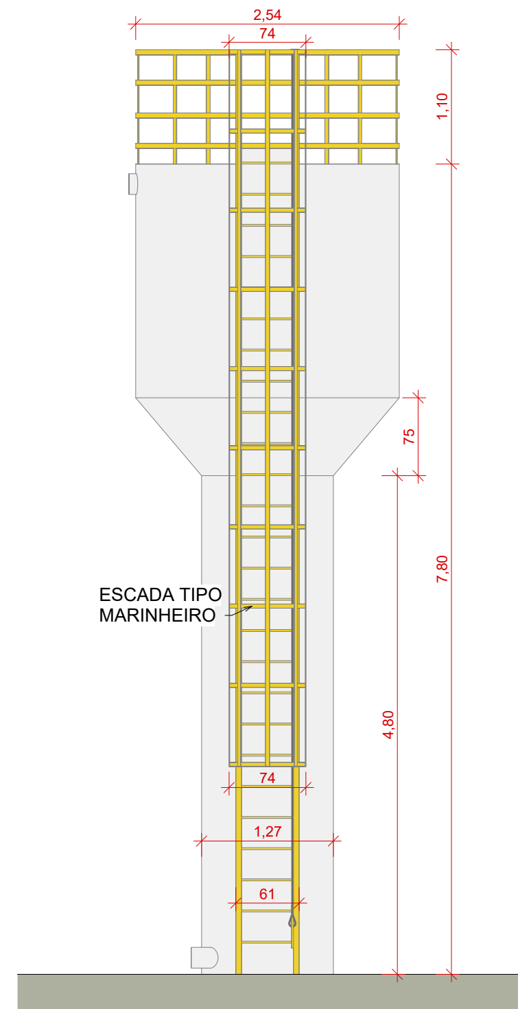
1 ELEVÇÃO FUNDO 1 : 50
