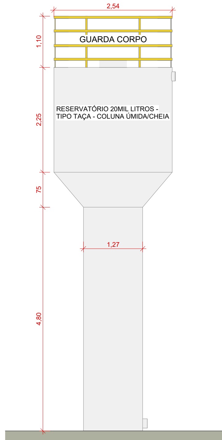
3 ELEVÇÃO FRONTAL 1 : 50
